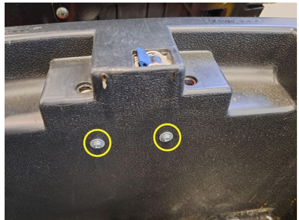
Irrota päävirtakytkimen kaksi kiinnitysruuvia. (ristipäämeisseli ph2).
