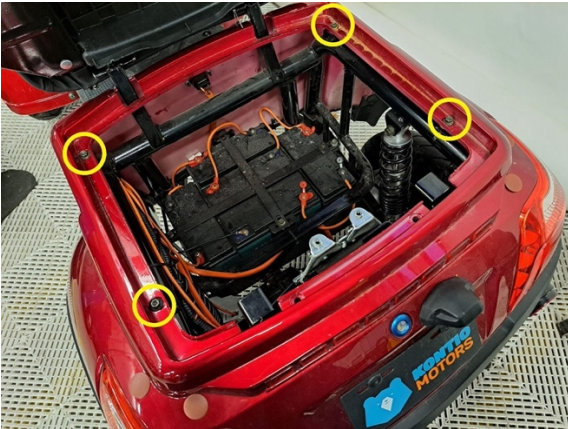
Irrota takakatteen neljä kiinnityspulttia. (hylsy 8 mm).
